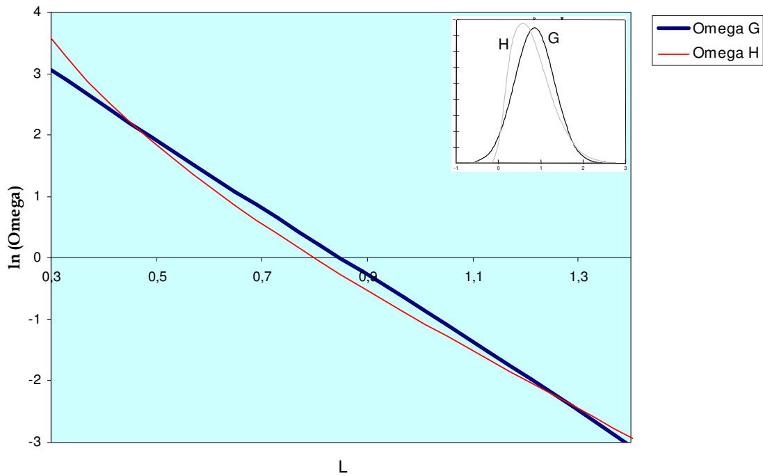
Figura 16 – Caso 4: Função \ln(\Omega(L)) para os ativos G e H
