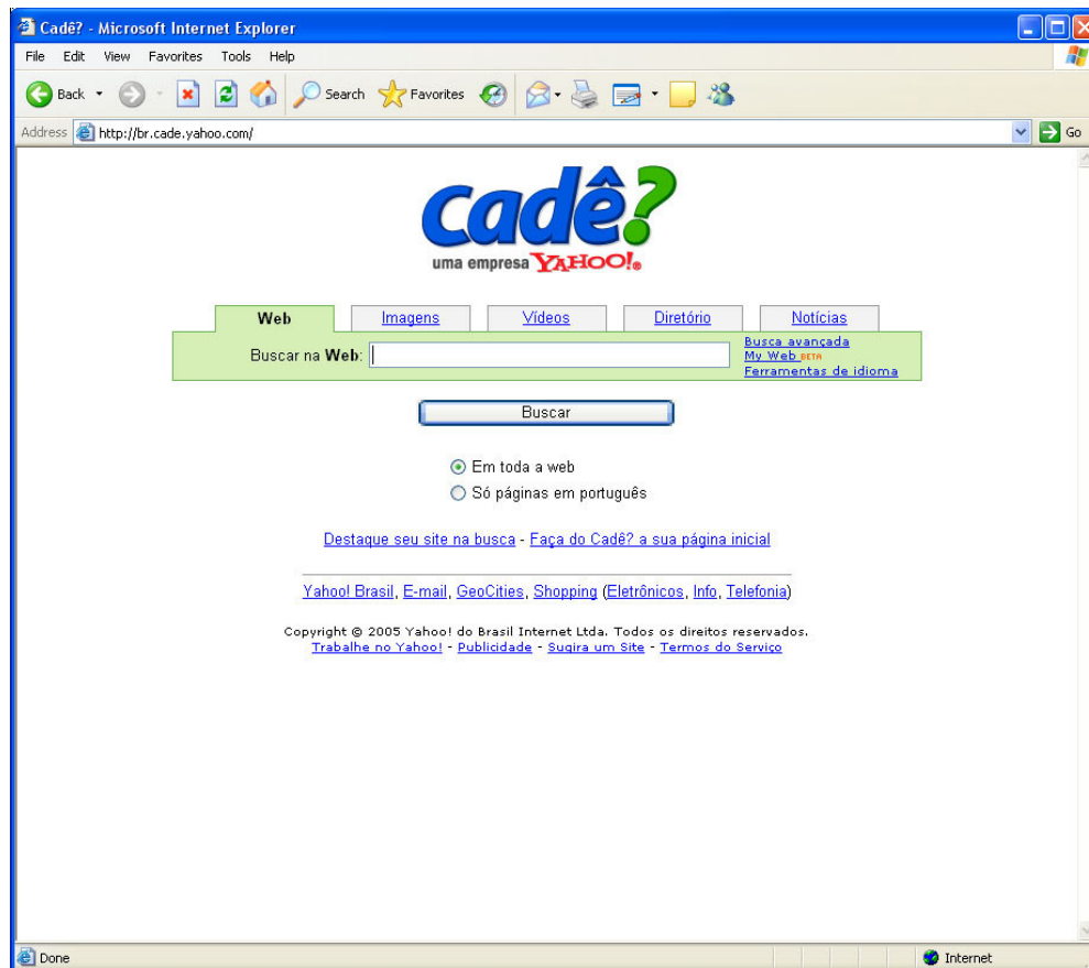
Figura 4 – Cadê (20/09/2006) http://www.cade.com.br
