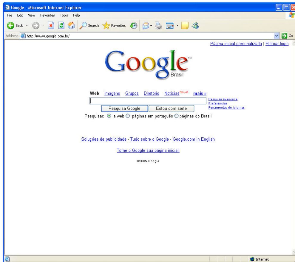
Figura 2 – Google (01/02/2007) http://www.google.com.br
