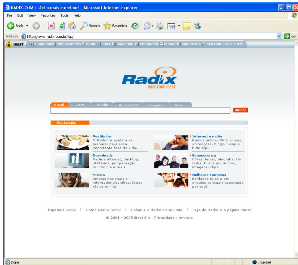
Figura 7 – Radix (30/06/2006) http://www.radix.com.br
