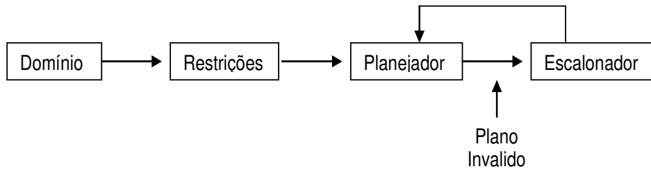
Figura 10 - Arquitetura com acoplamento fraco
