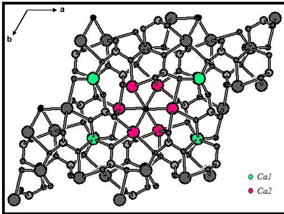
Figura 2.2.1A Célula unitária (2,2,1) em projeção paralela ao plano a,b, indicando os sítios 1 e 2 do cálcio.
