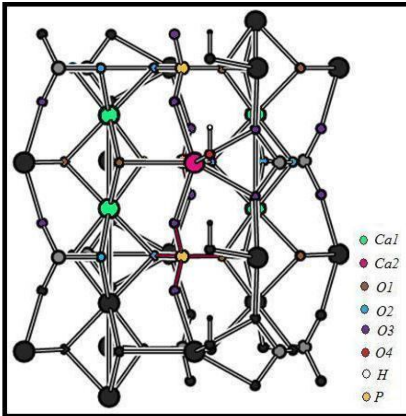
Figura 2.2.2 Célula unitária (1,1,2) vista ao longo da direção c indicando a vizinhança e os planos cristalinos onde se situam Ca1, Ca2, O1, O2, O3, O4, P e H. O4 é o oxigênio da hidroxila.
