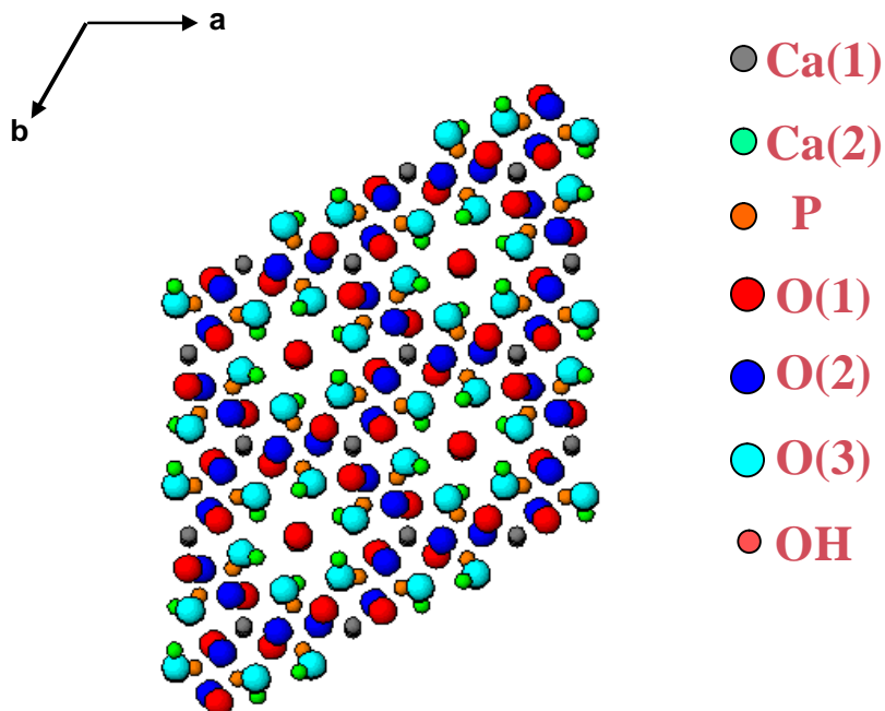
Figura 2.2.1B Célula unitária (2,2,1) em projeção paralela ao plano a,b, indicando os átomos de sua composição
