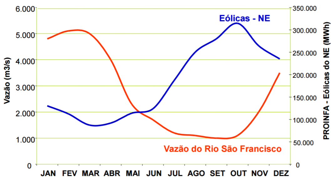
Gráfico 4 – Exemplo de complementaridade sazonal entre os ventos e as vazões hídricas. Fonte: CEPEL.
